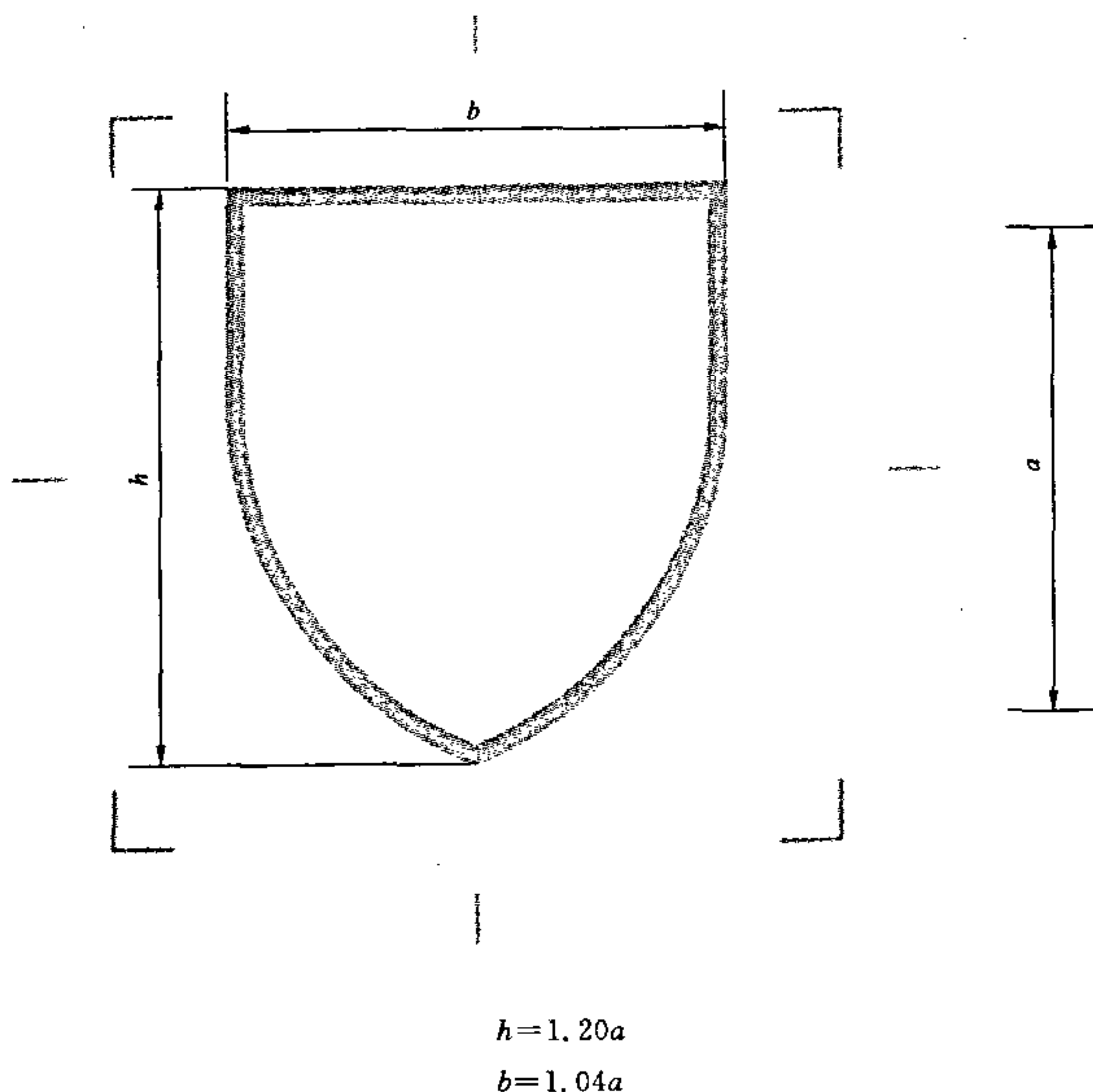
图 B.1 ISO 7000-2410 防护的基本图形符号
